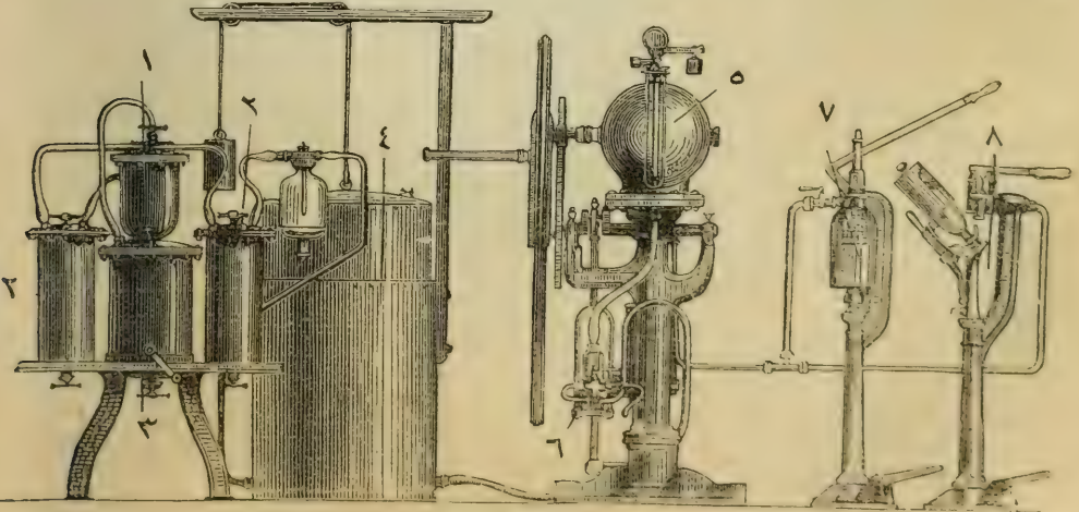
غازوز ماكنهسى ۱ - حافى محفوظى ، ۲ - مفصل ، ۳ - حاص قاربون مرلدى ، ۴ - مقياس غاز ، ۵ - مكشفه ، ۶ - طنزويه ، ۷ و ۸ - غازك شينه و سينونه ملاسه مخصوص الات .
